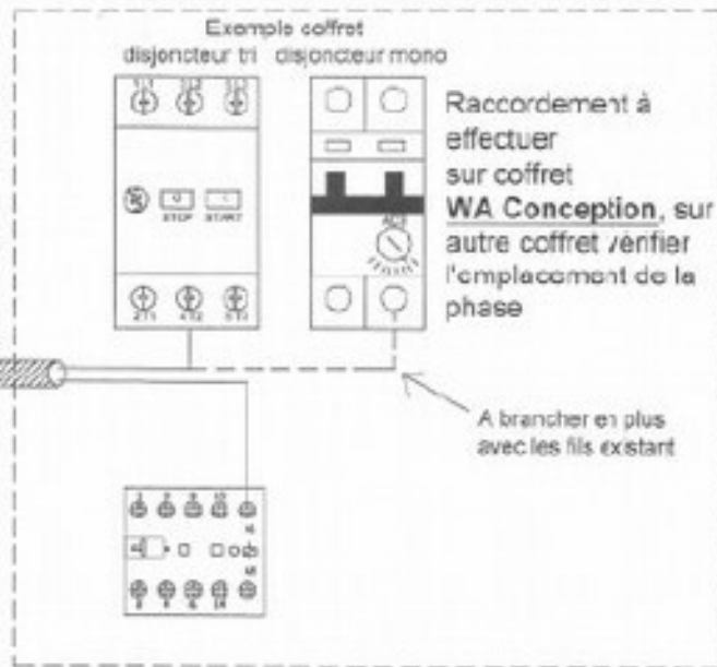
COFFRET ELECTRIQUE DE FILTRATION
